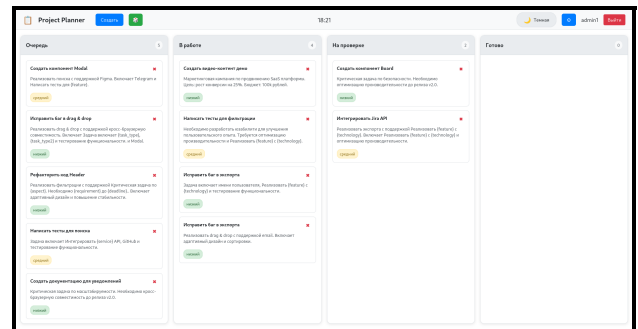
Рис. 4: Светлая тема
