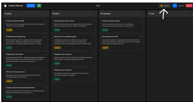
Рис. 3: Темная тема
